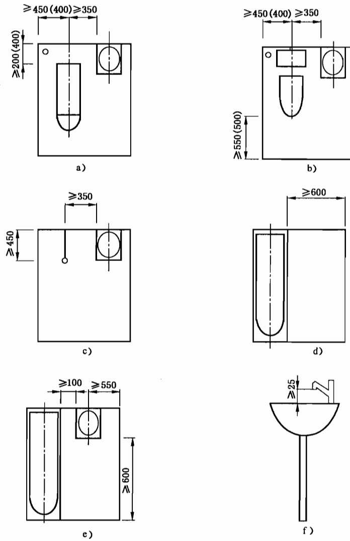
图 1 卫生间配套设备安装示意图
